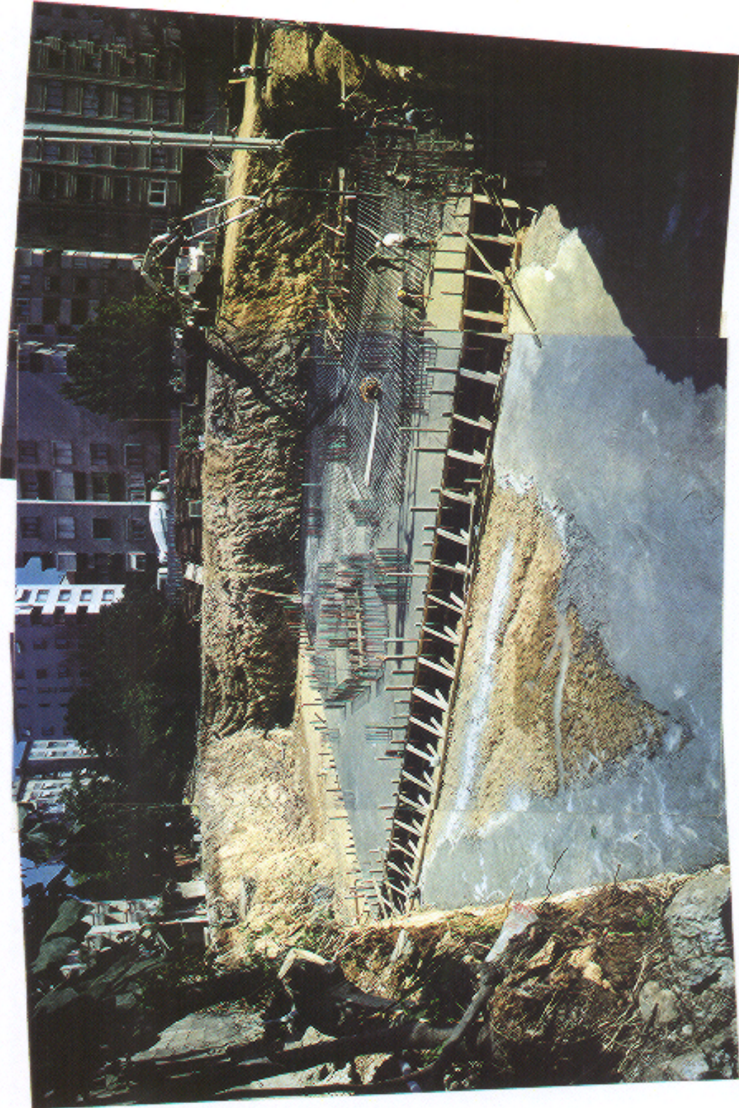
Temizlik betonu, donatılar ve B 25 Temel dökümü
